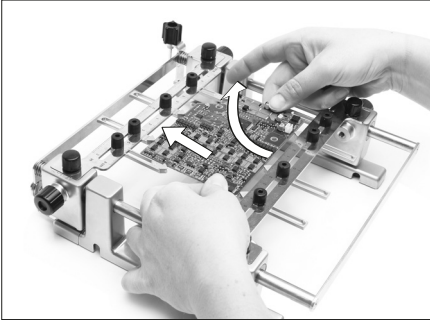
取下PCB板
